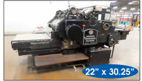
ORIGINAL HEIDELBERG SBGS DIE CUTTER
